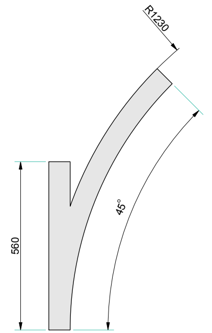
Y Bends
